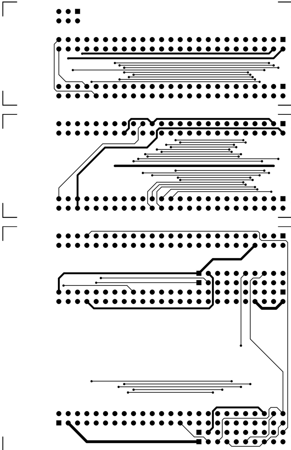
Top Layer
