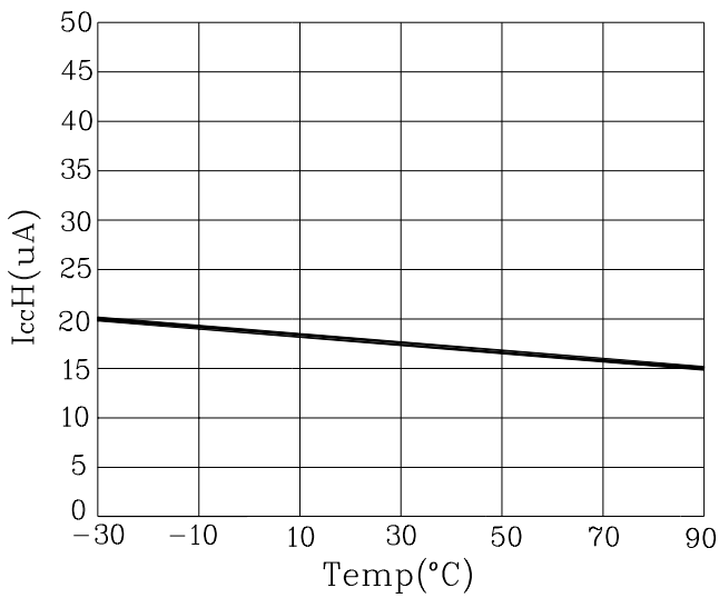
Fig. 3 I_{CCH} - Temp
