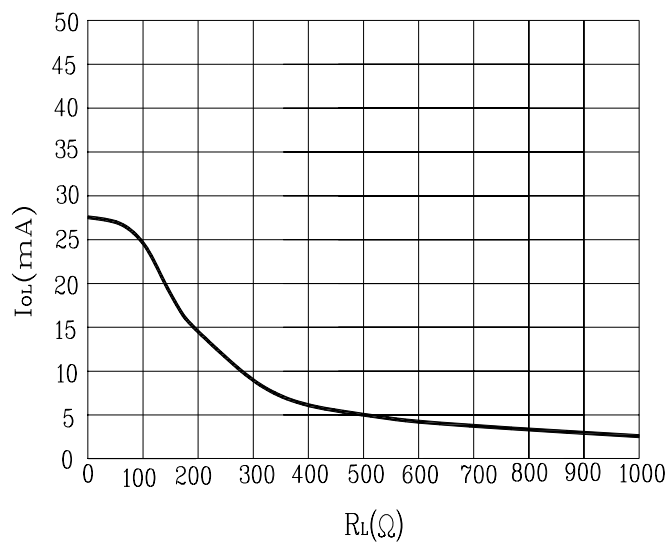
Fig. 4 I_{OL} - R_L
