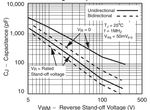
Fig. 6 - Capacitance
