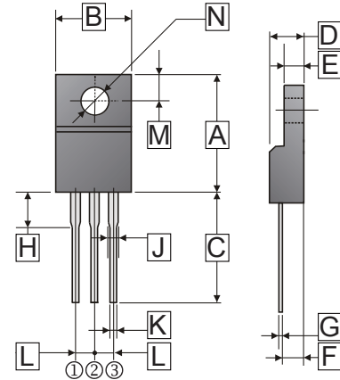
ITO-220
