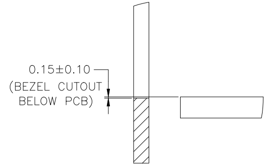
DETAIL K 2:1
