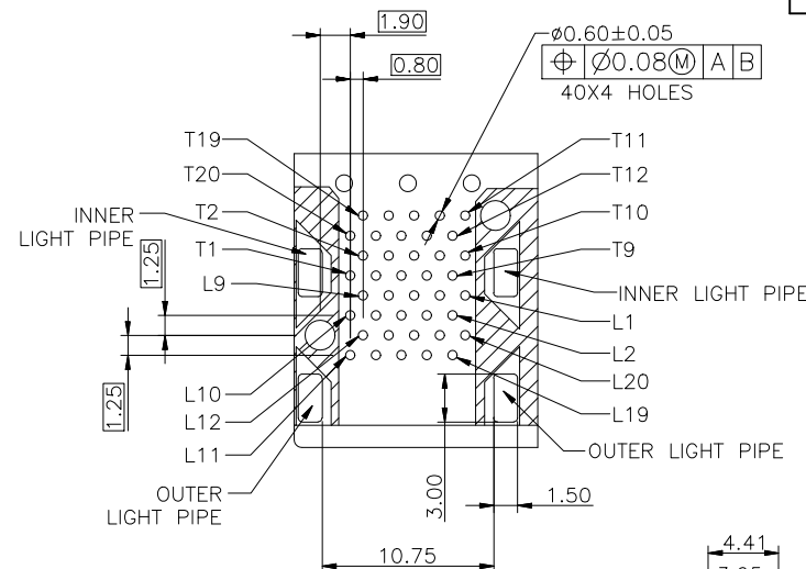
DETAIL H 2:1
