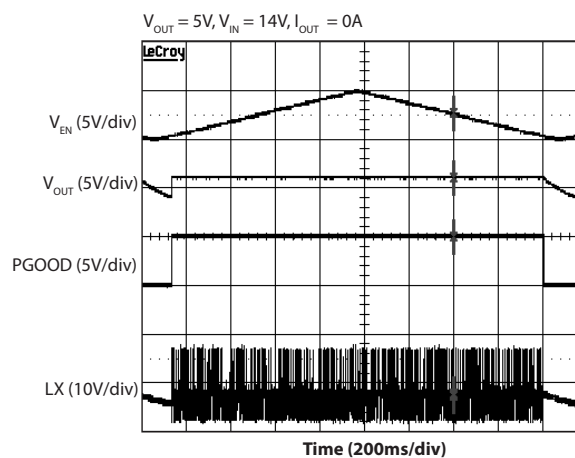
EN Ramp
