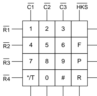
SC9302G
