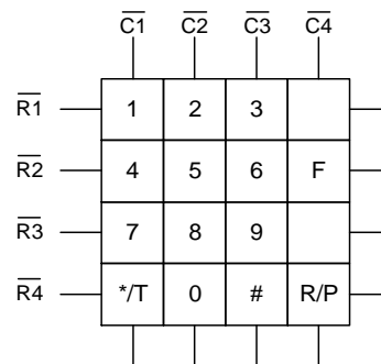
SC9302H
