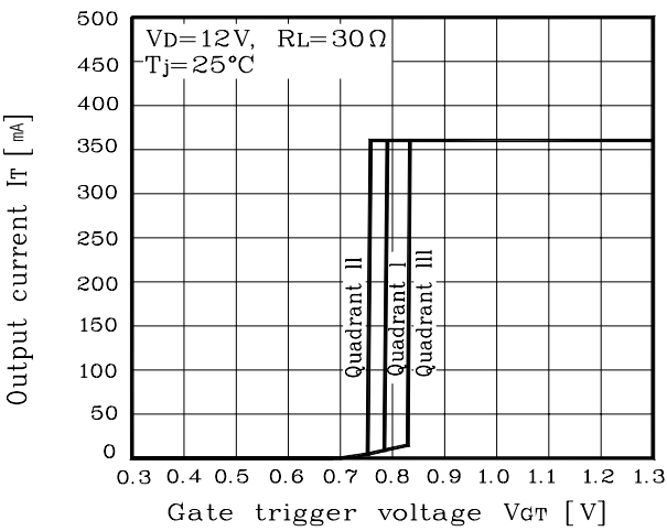
Fig. 8 I_T - V_{GT}
