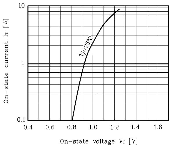
Fig. 3 I_T - V_T
