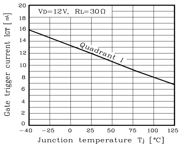
Fig. 5 I_{GT} - T_j
