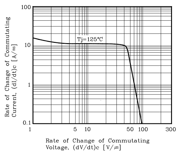
Fig. 4 (di/dt)_c - (dV/dt)_c
