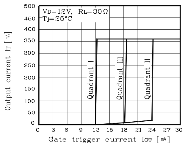
Fig. 6 I_T - I_{GT}
