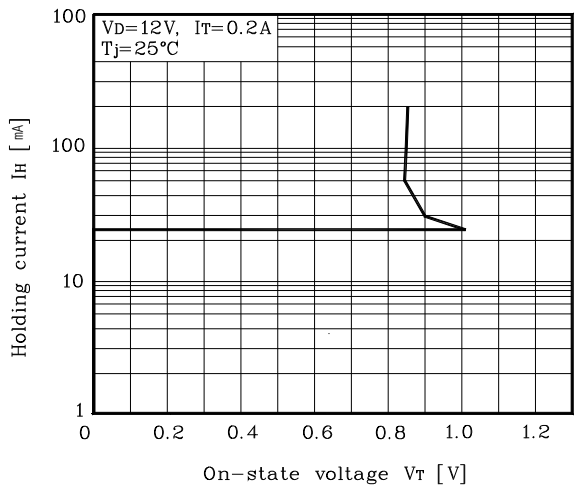
Fig. 9 I_H - V_T
