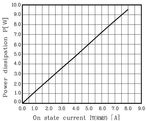
Fig. 1 P - I_{T(RMS)}
