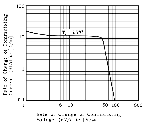
Fig. 4 (dI/dt)_C - (dV/dt)_C
