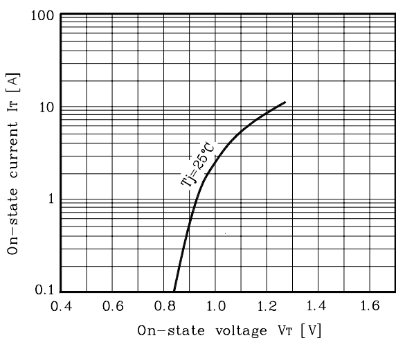
Fig. 3 I_T - V_T
