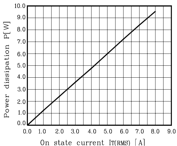
Fig. 1 P - I_{T(RMS)}
