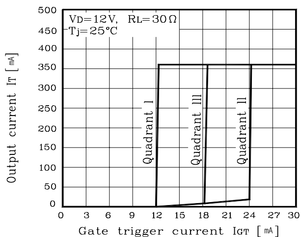
Fig. 6 I_T - I_{GT}
