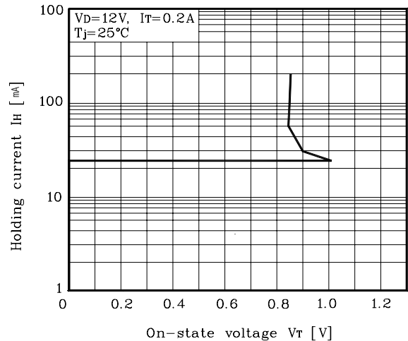
Fig. 9 I_H-V_T
