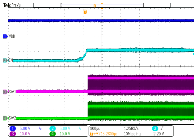
Figure 14. EN Startup
