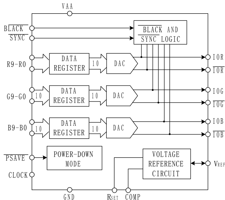
图 1 原理框图:
