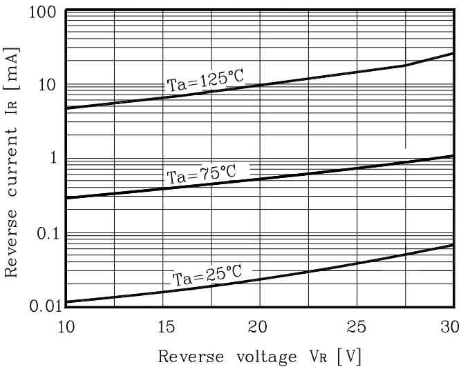
Fig. 2 I_R - V_R
