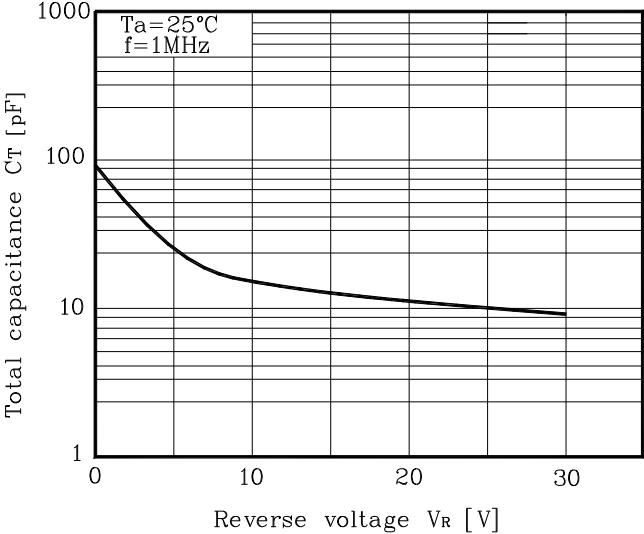
Fig. 3 C_T - V_R
