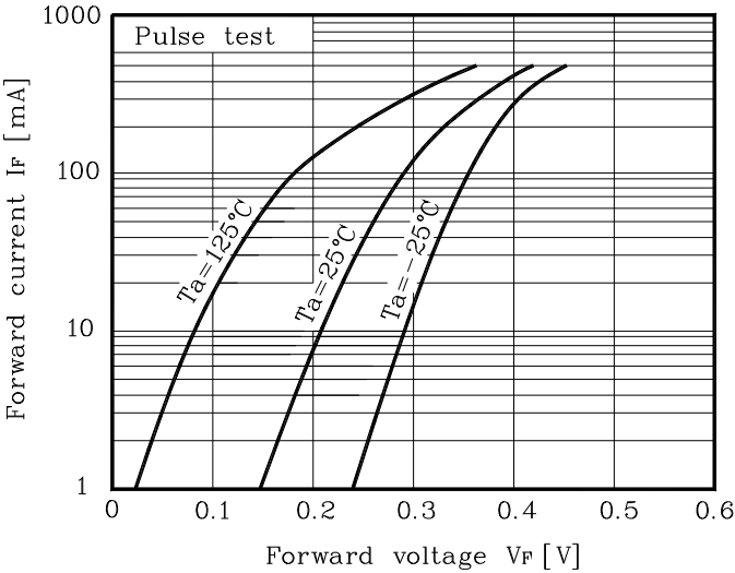
Fig. 1 I_F - V_F
