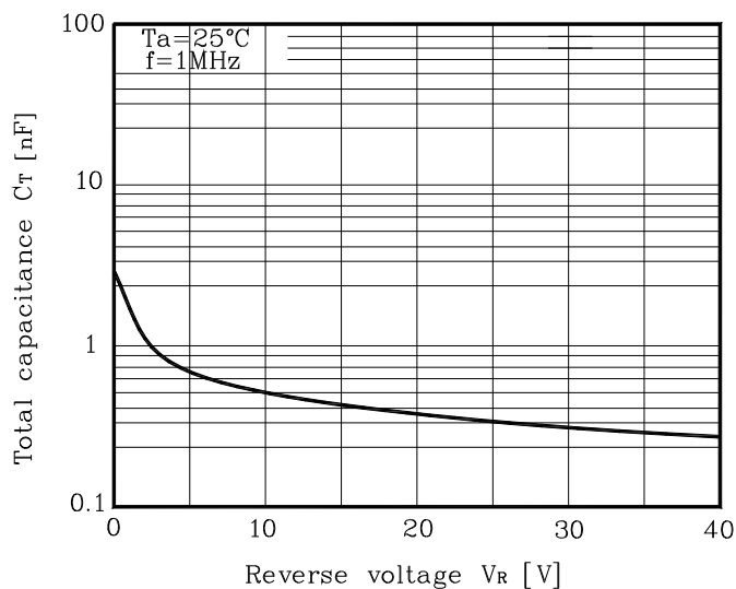
Fig. 4 C_T - V_R
