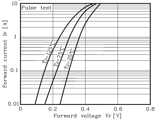
Fig. 1 I_F - V_F
