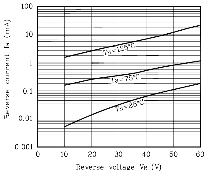
Fig. 2 I_R - V_R
