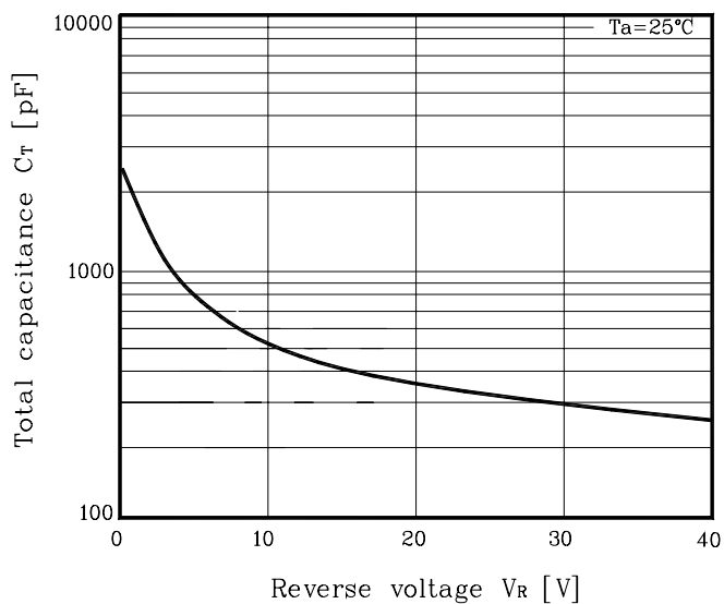
Fig. 3 C_T - V_R
