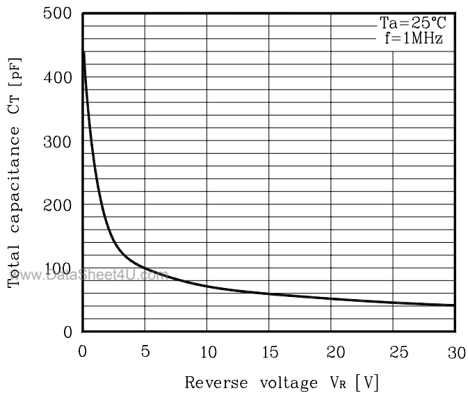
Fig. 3 C_T - V_R
