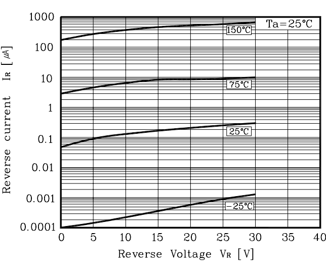
Fig. 2 I_R - V_R
