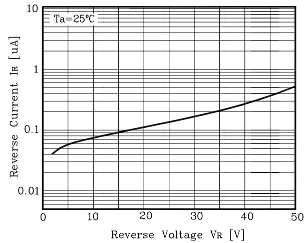
Fig. 2 I_R - V_R
