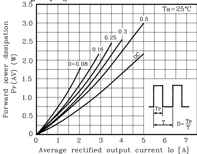
Fig. 3 P_F - I_O
