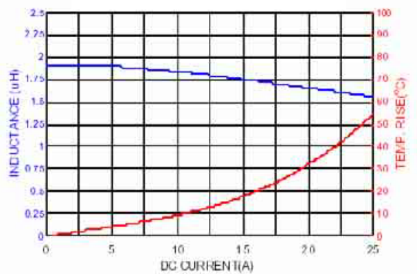
SDL1108-2R0MF
