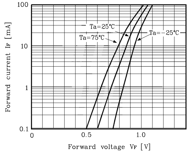
Fig. 2 I_F - V_F
