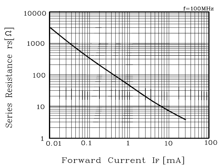
Fig. 4 r_s - I_F
