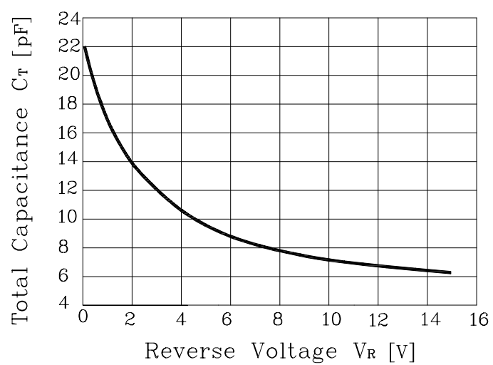
Fig. 1 C_T - V_R
