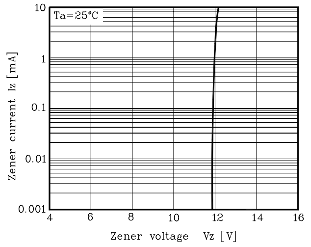
Fig. 2 I_Z.V_Z
