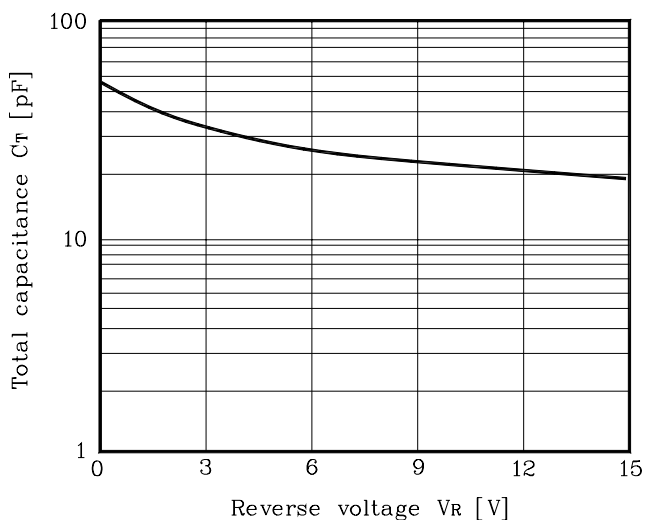
Fig. 3 C_T - V_R
