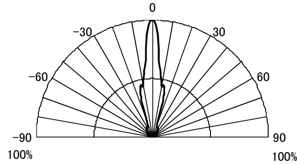
指向特性図
