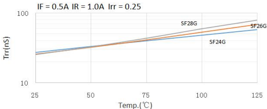
Fig.5 Trr & Temp.
