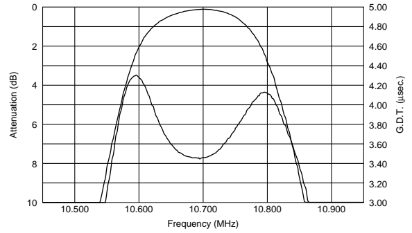
SF ECS10M7GA00-R0
