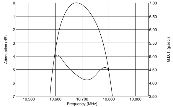
SFELA10M7JAB0-B0
