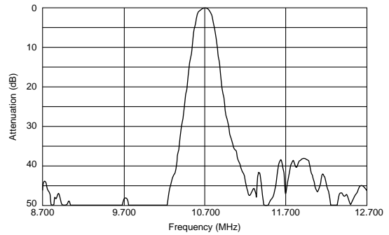
SF ECS10M7GA00-R0
