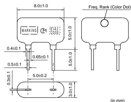
CDALA10M7G_Series
