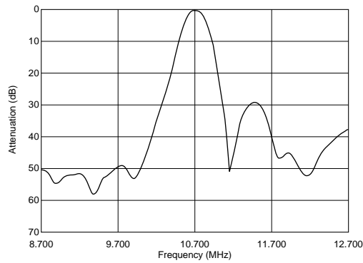
SFELA10M7GAXX-B0
