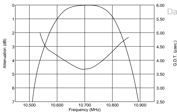
SFTLA10M7FA00-B0
