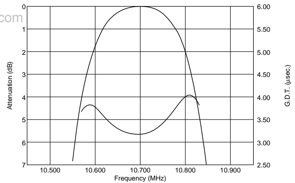
SFELA10M7GAB0-B0
