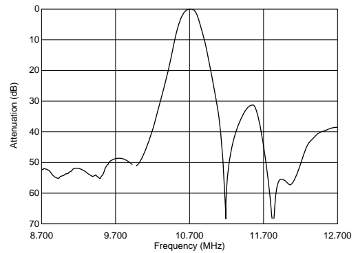
SFELA10M7GAXA-B0
