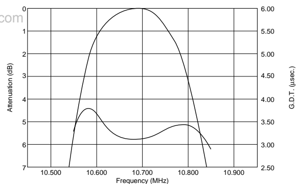
SFELA10M7GA0G-B0
