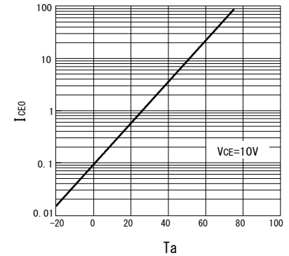
■ 暗電流/周囲温度特性 I_{CE0} (nA) / T_a (°C)
