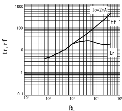
■ 応答時間/負荷抵抗特性 *1 t_r, t_f ( \mu\text{sec} ) / R_L ( \Omega )
