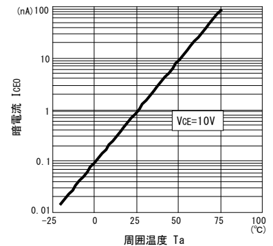
■ 暗電流/周囲温度特性 I_{CE0}/T_a
