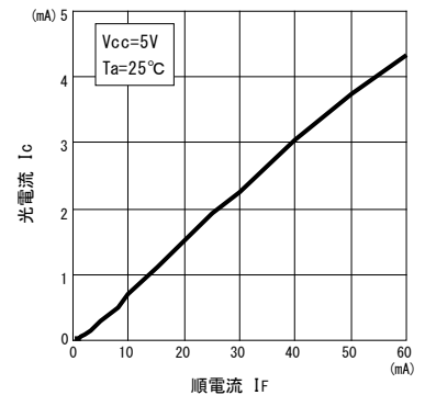
■ 光電流/順電流特性 I_C/I_F
