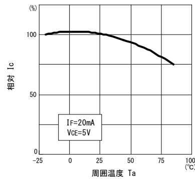
■ 相対光電流/周囲温度特性 相対 I_C/T_a
