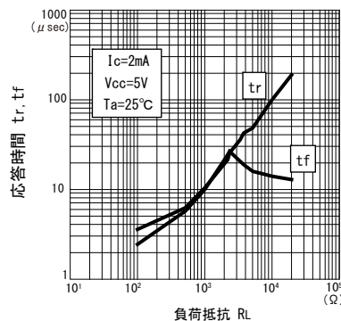
■ 応答時間/負荷抵抗特性 *1 t_r, t_f (\mu\text{sec})/R_L
