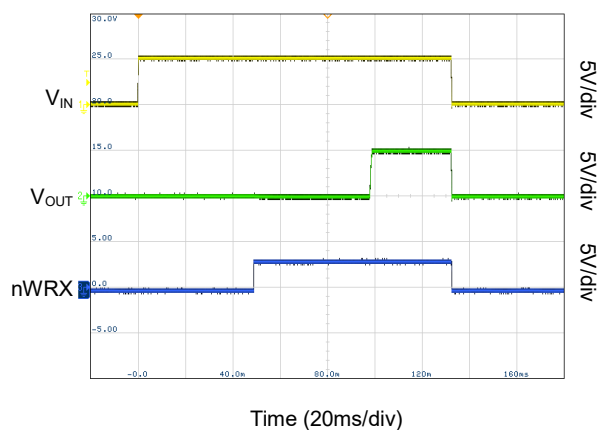
VIN 5V Insert-Remove
