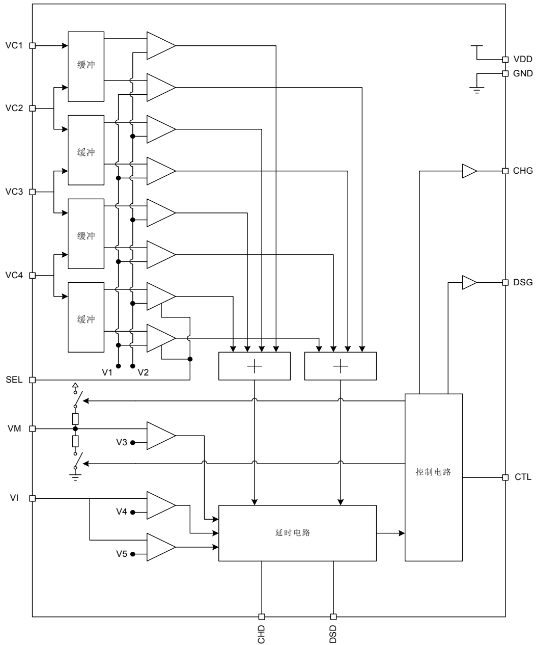
图1 SH367003系统框图
