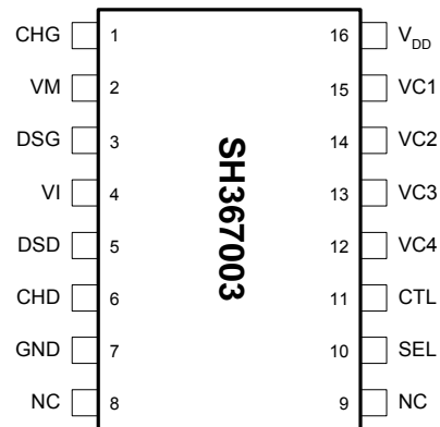
图2 SH367003引脚配置图
