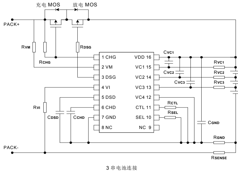
3 串电池连接
