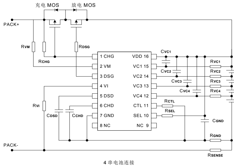
4 串电池连接
