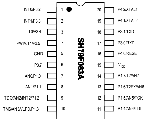
引脚配置图
