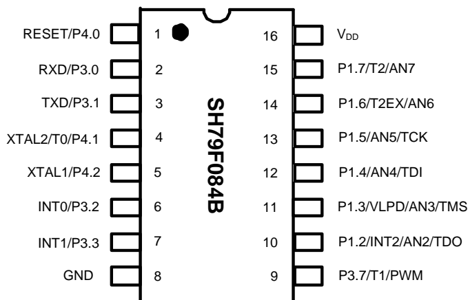
引脚配置图
