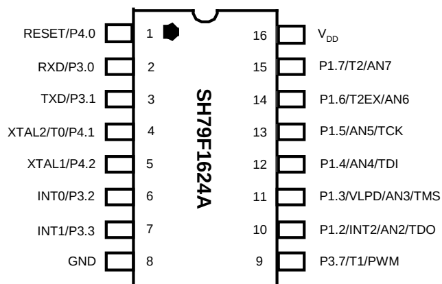
引脚配置图
