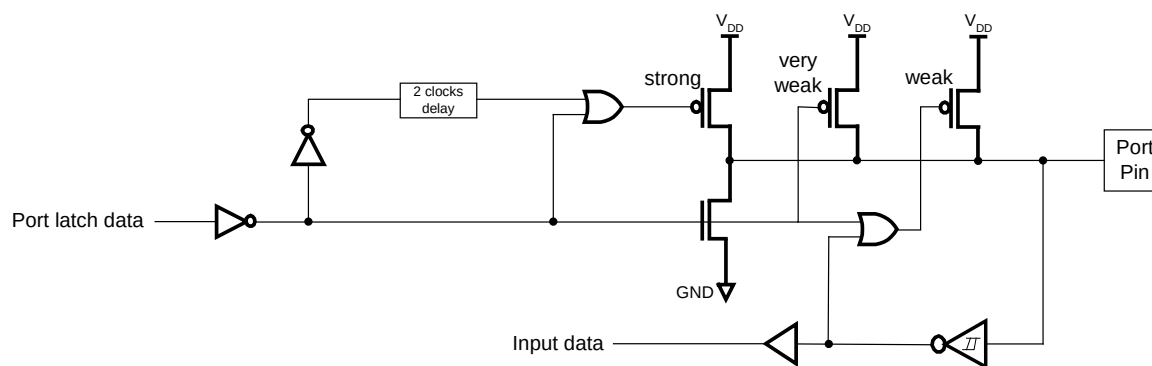
准双向结构
