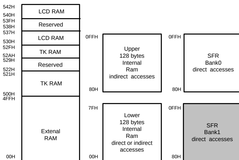
内部和外部RAM配置
