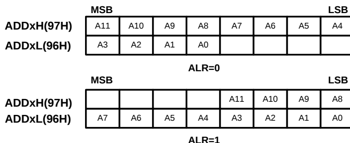
图9.8-3 ADC转换结果存储方式示意图
