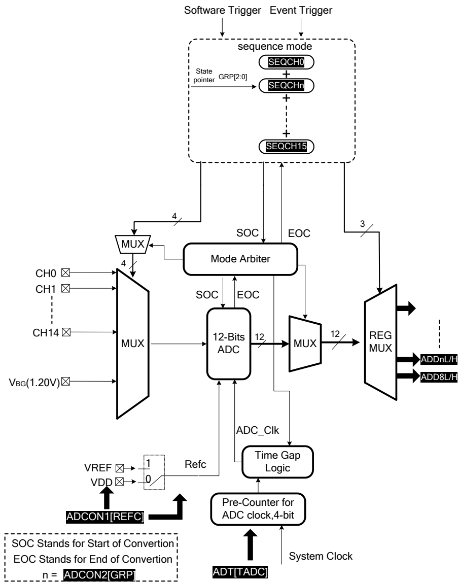
图8.8-1 ADC模块图
