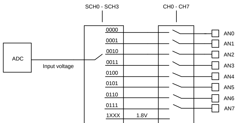
AD转换器模块图
