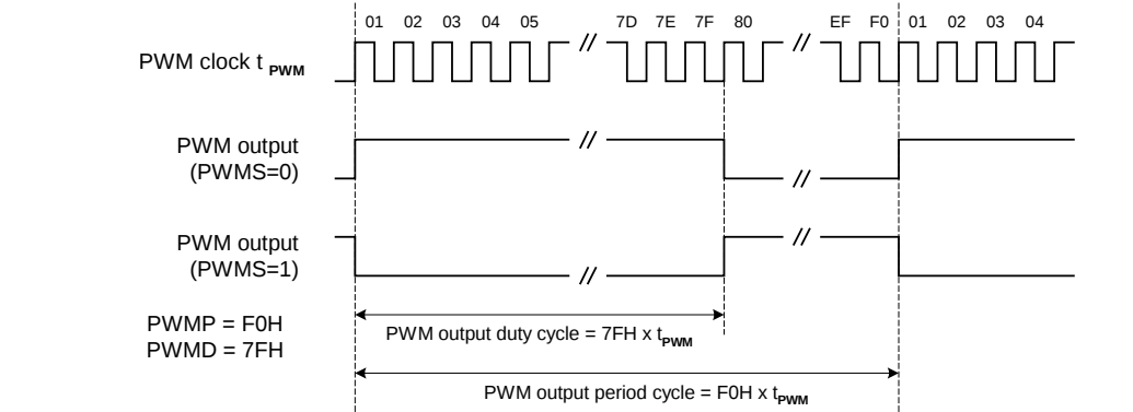
PWM 输出示例
