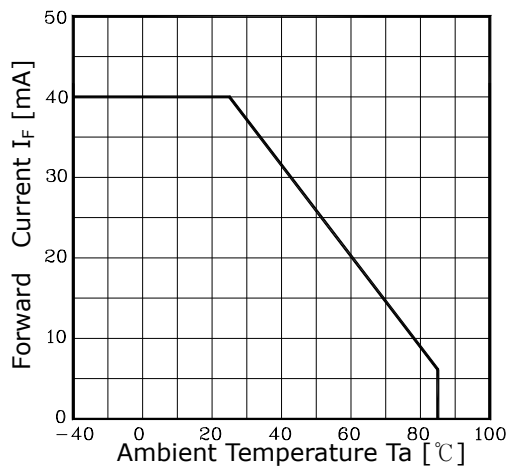
Fig. 3 I_F - T_a
