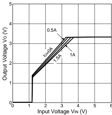
Output Voltage(SI-3033C)
