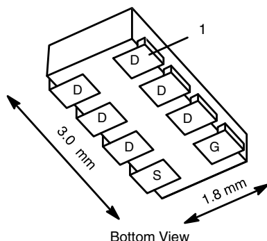
ChipFET 1206-8
