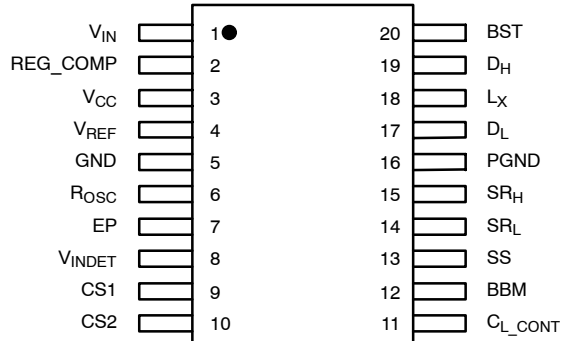
Si9122DQ (TSSOP-20)
