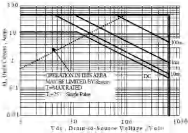
图 6-3 SIF12N65F(TO-262&263)
