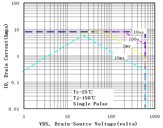
图 6-2 SIF2N60D (TO-220FP)
