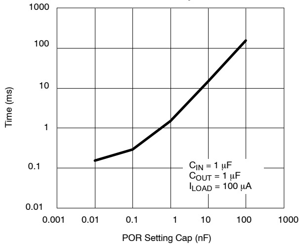
POR Delay
