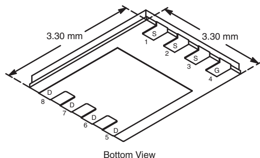
PowerPAK 1212-8
