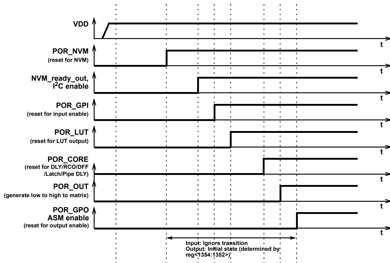
Figure 77. POR sequence
