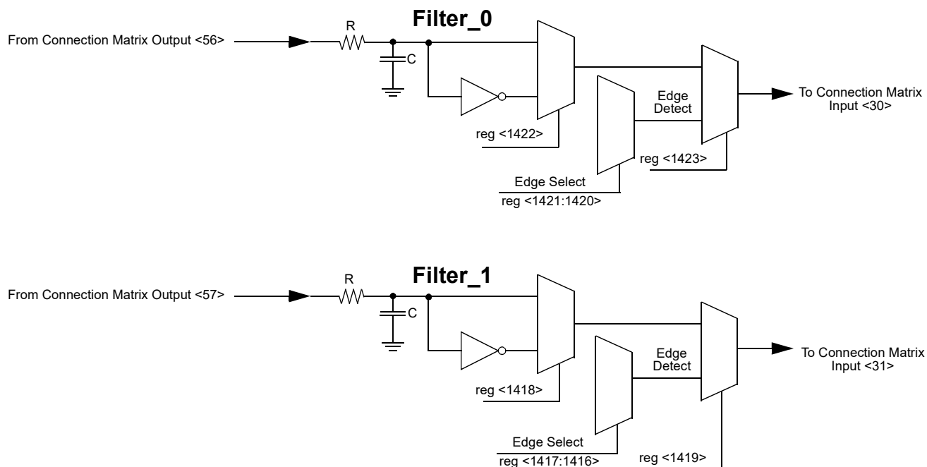
Figure 44. Deglitch Filter / Edge Detector
