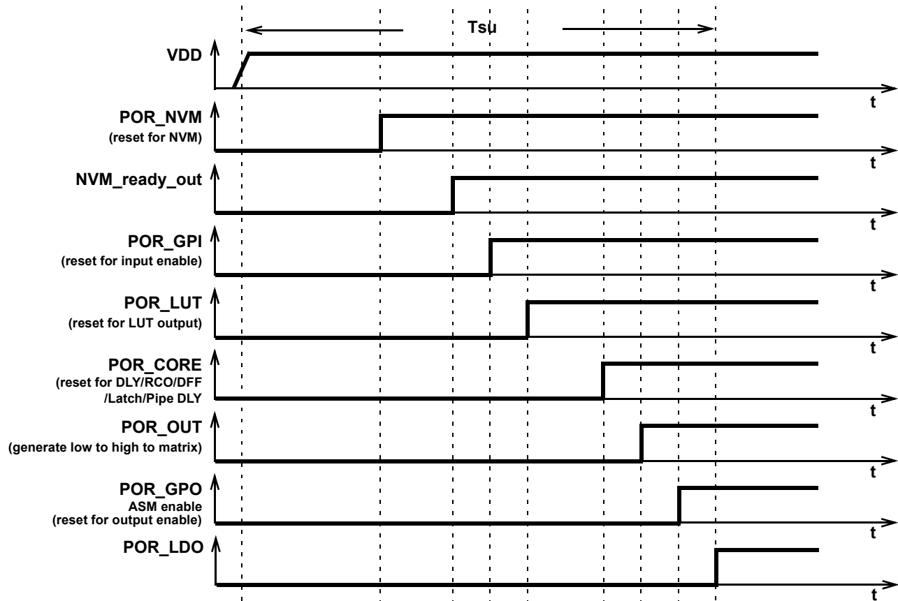
Figure 54. POR sequence
