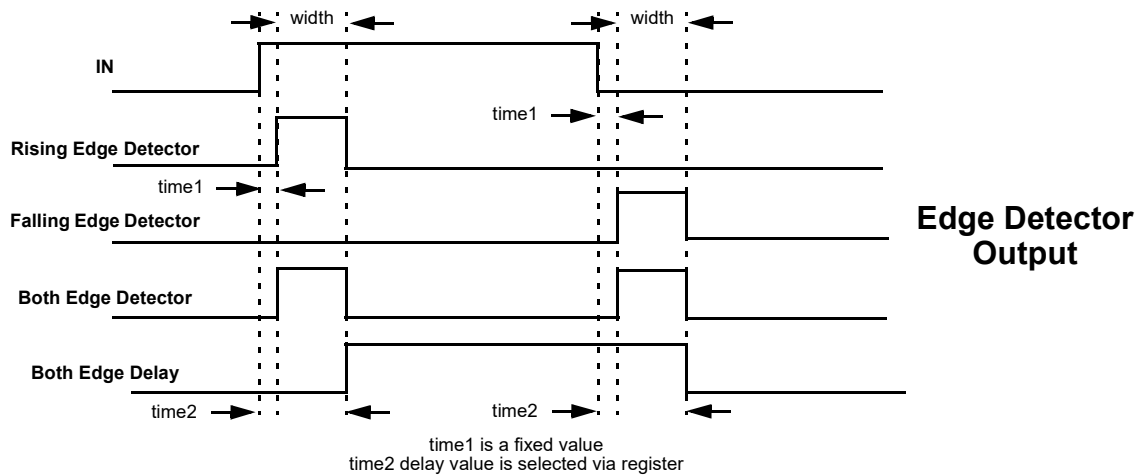
Figure 43. Edge Detector Output
